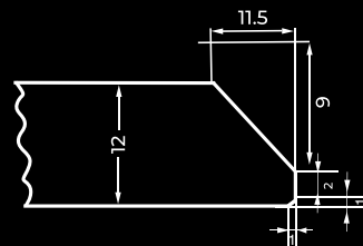
ФРЕЗЕРУВАННЯ ФАСКИ F-TOUCH
