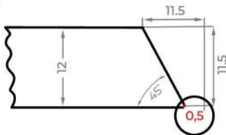
ЗРІЗ ПІД 45°
