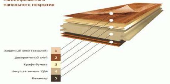
Основные составляющие ламинированного напольного покрытия
